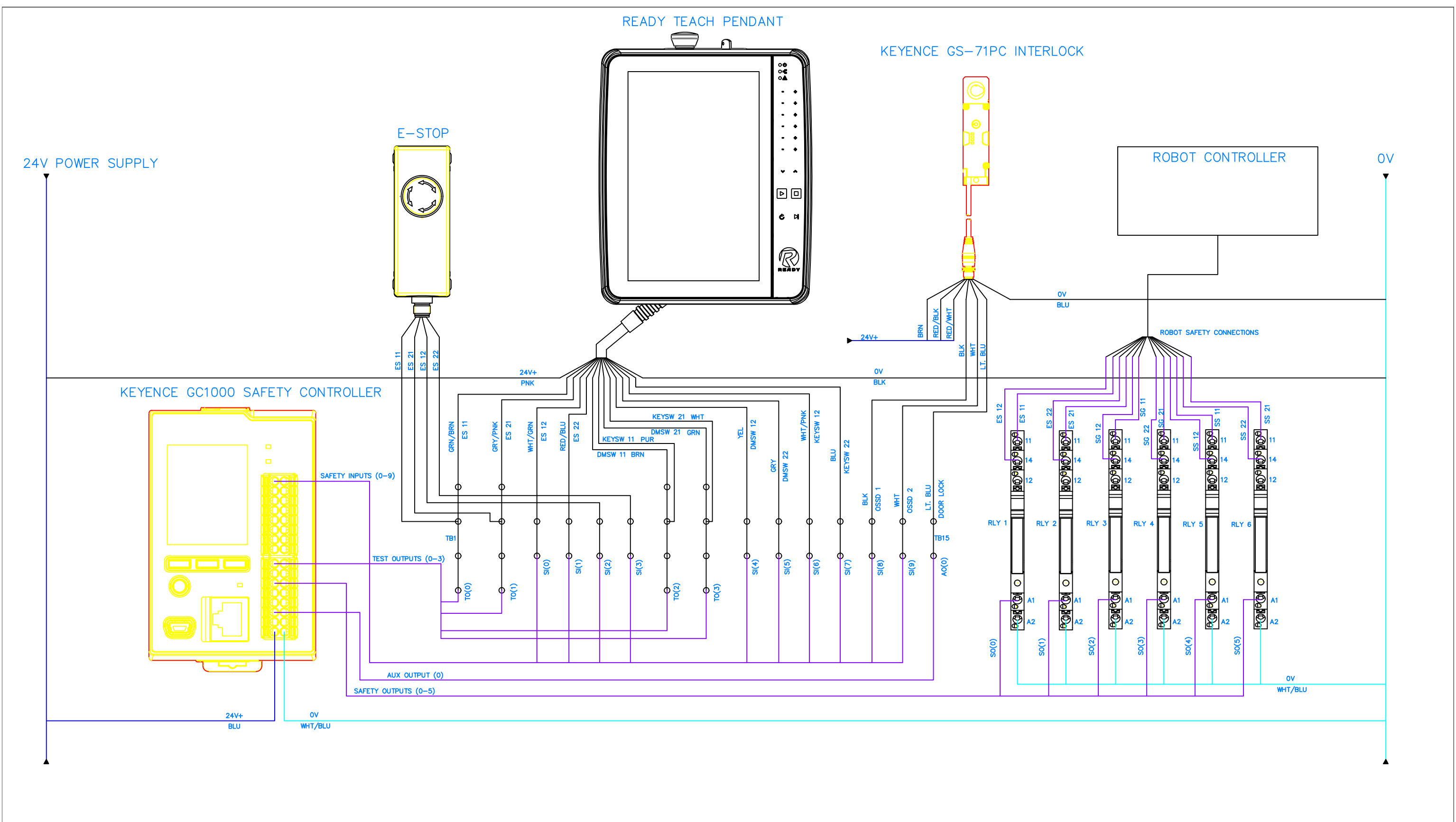
GC1000 Wiring Example
